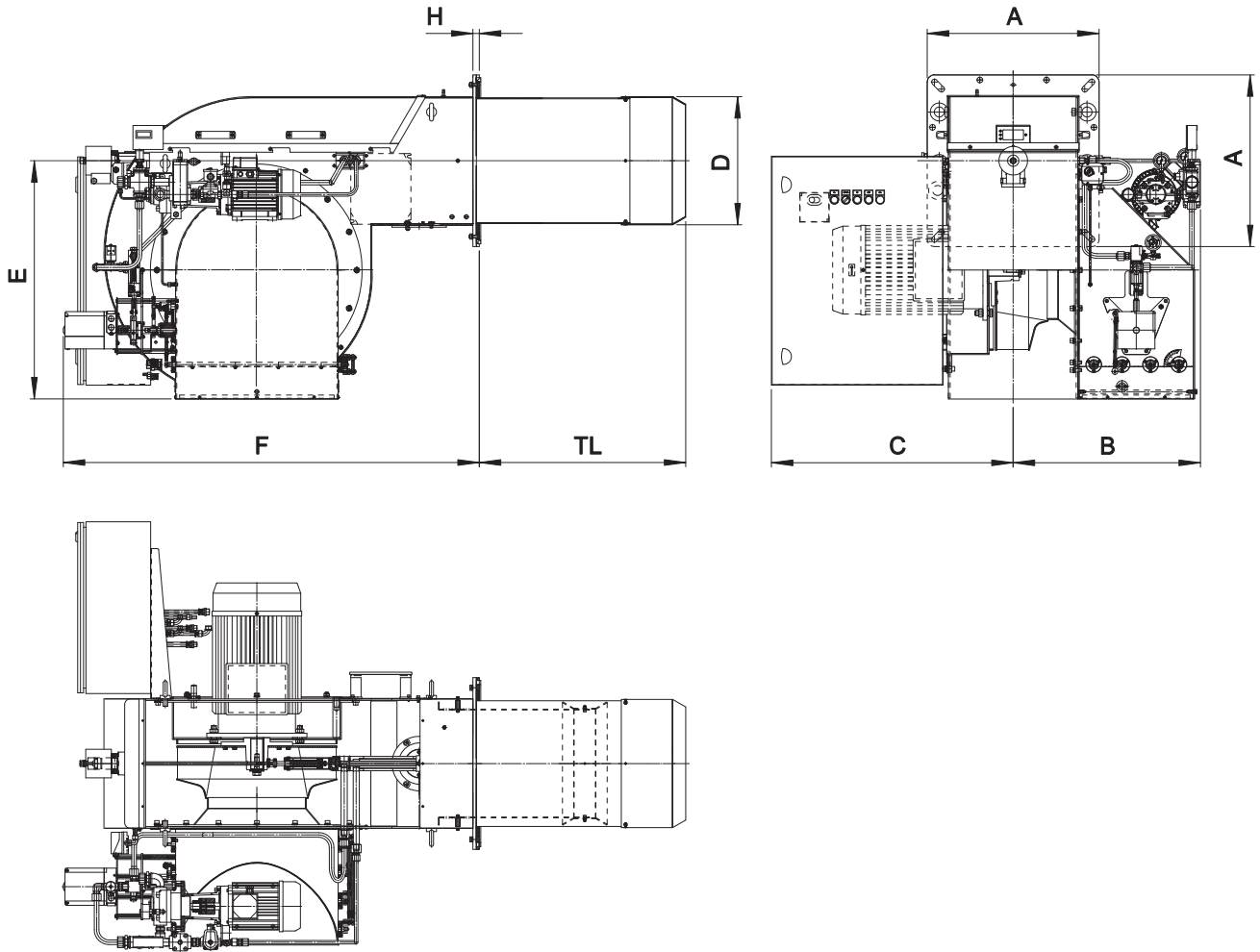
Fig. 2 Dimensions
