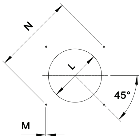
Fig. 3 Plaque porte-brûleur
