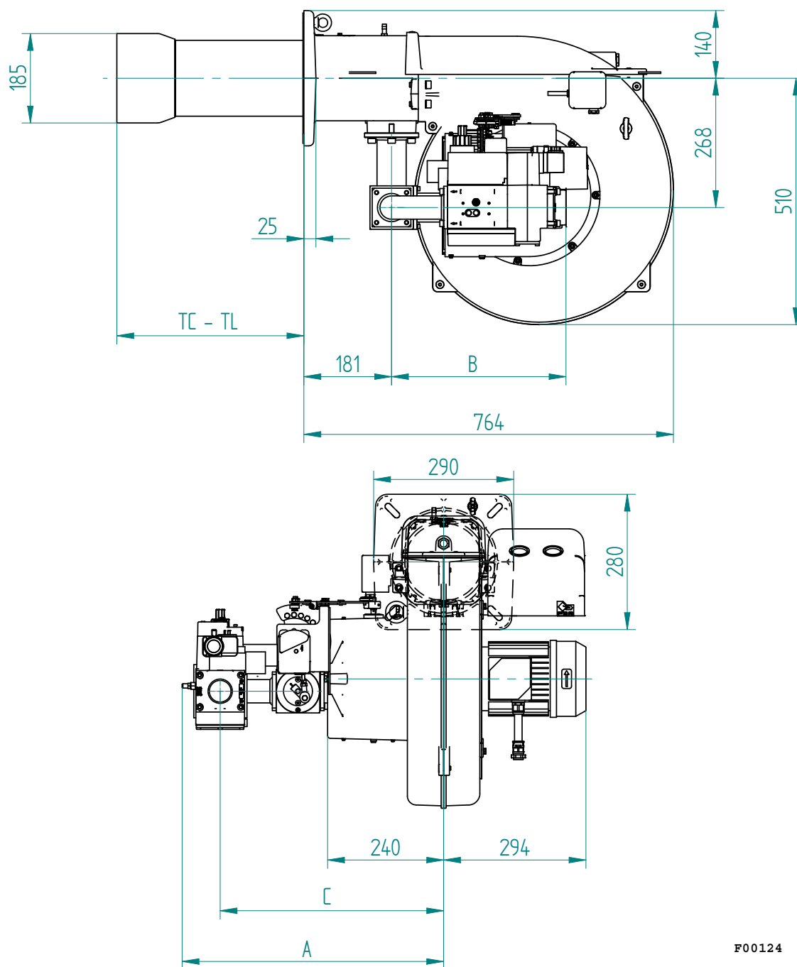
Fig. 3 Dimensioni ingombro
