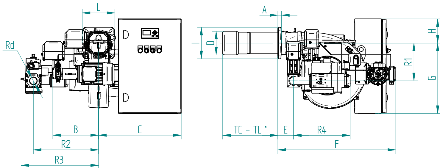
Fig. Dimensions
