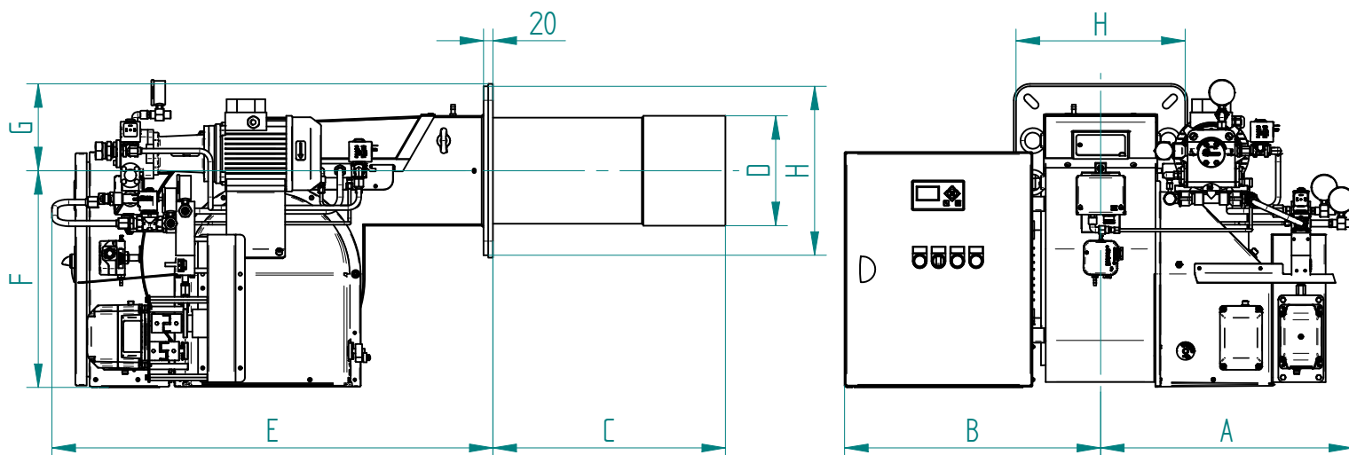
Fig. 4 Medidas FGP 190/M-EL - FGP 250/M-EL
