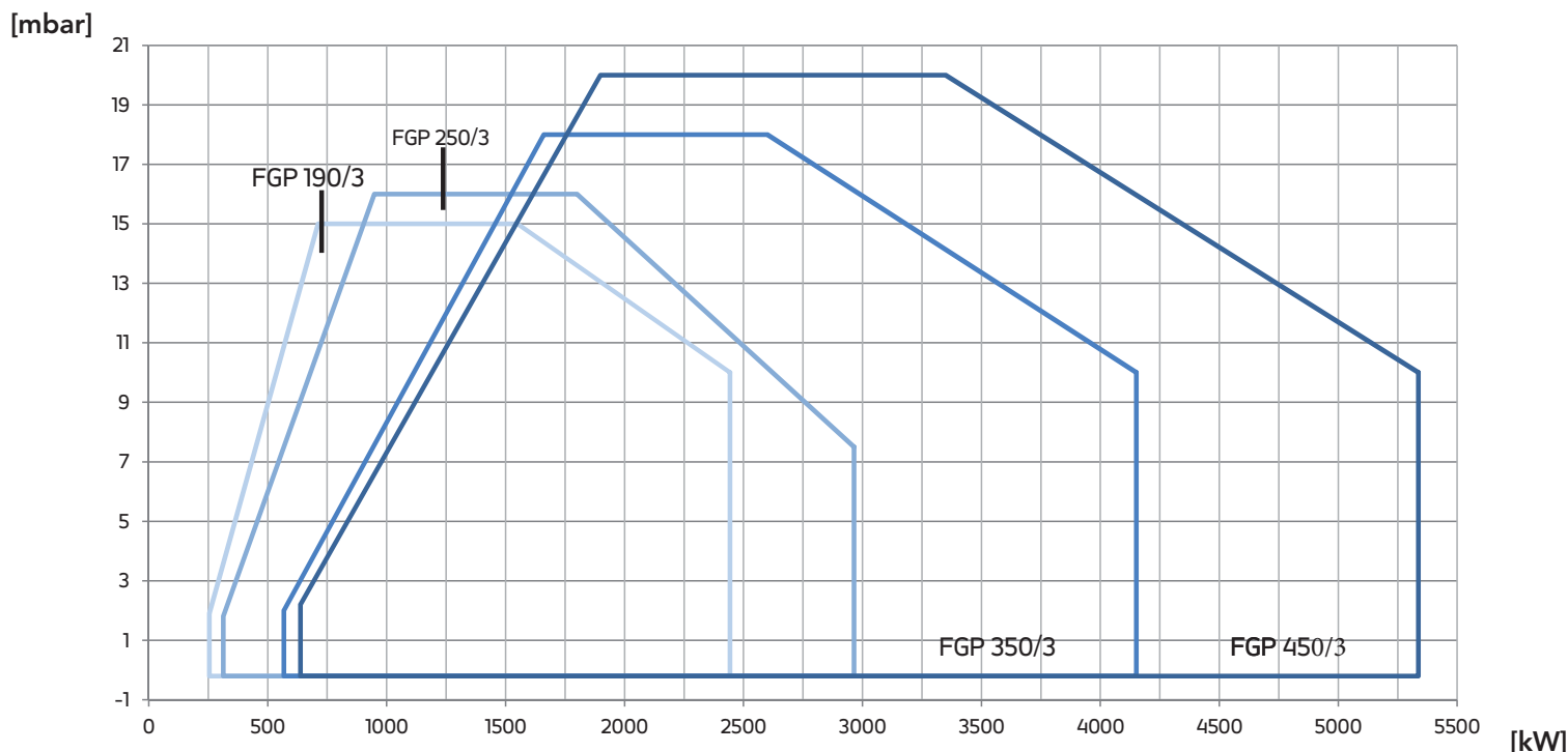
Fig. 2 X = Puissance Y = Pression à la chambre de combustion
