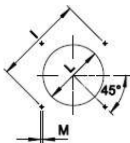
Fig. 4 Plaque porte-brûleur
