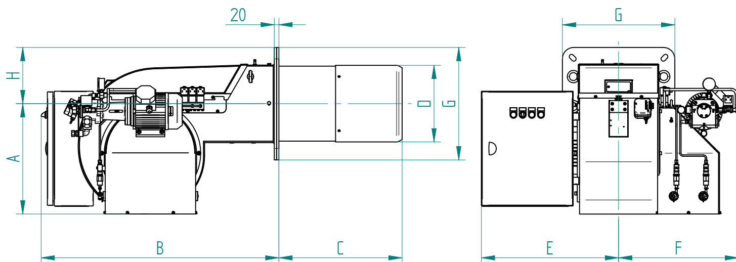
Fig. 3 Dimensioni FGP 190/3 - FGP 250/3 - FGP 350/3 - FGP 450/3
