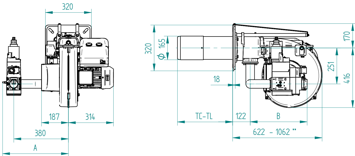
Fig. 3 Dimensions
