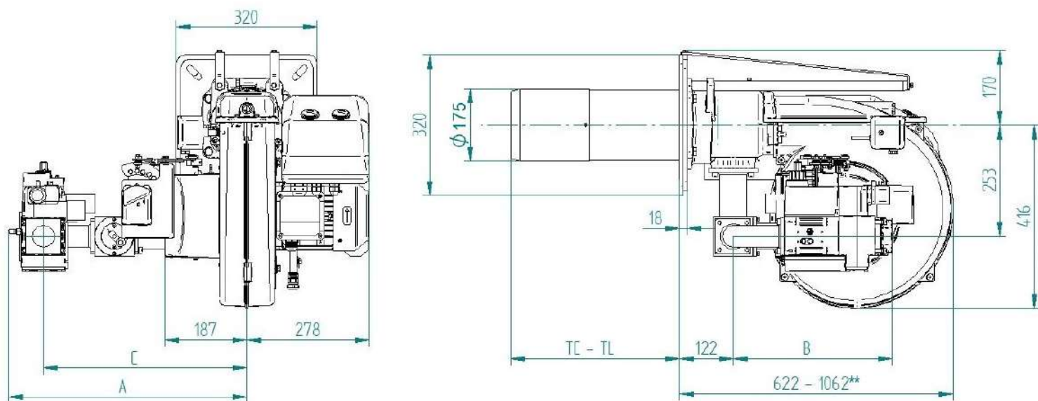
Fig. 3 Dimensioni ingombro
