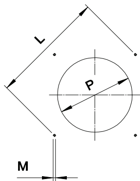
Fig. 3 Flangia fissaggio bruciatore
