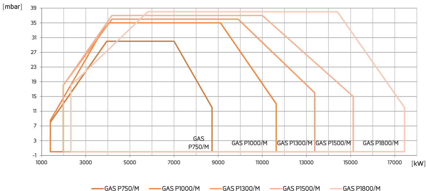
Fig. 1 X = Potenza termica Y = Pressione in camera di combustione (mbar)
