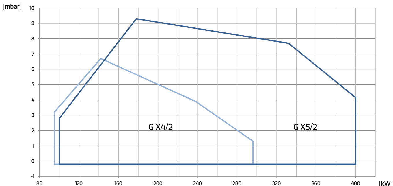
Fig. 3 X = Puissance Y = Pression en chambre de combustion
