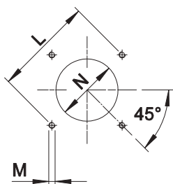
Fig. 9 Plaque porte-brûleur
