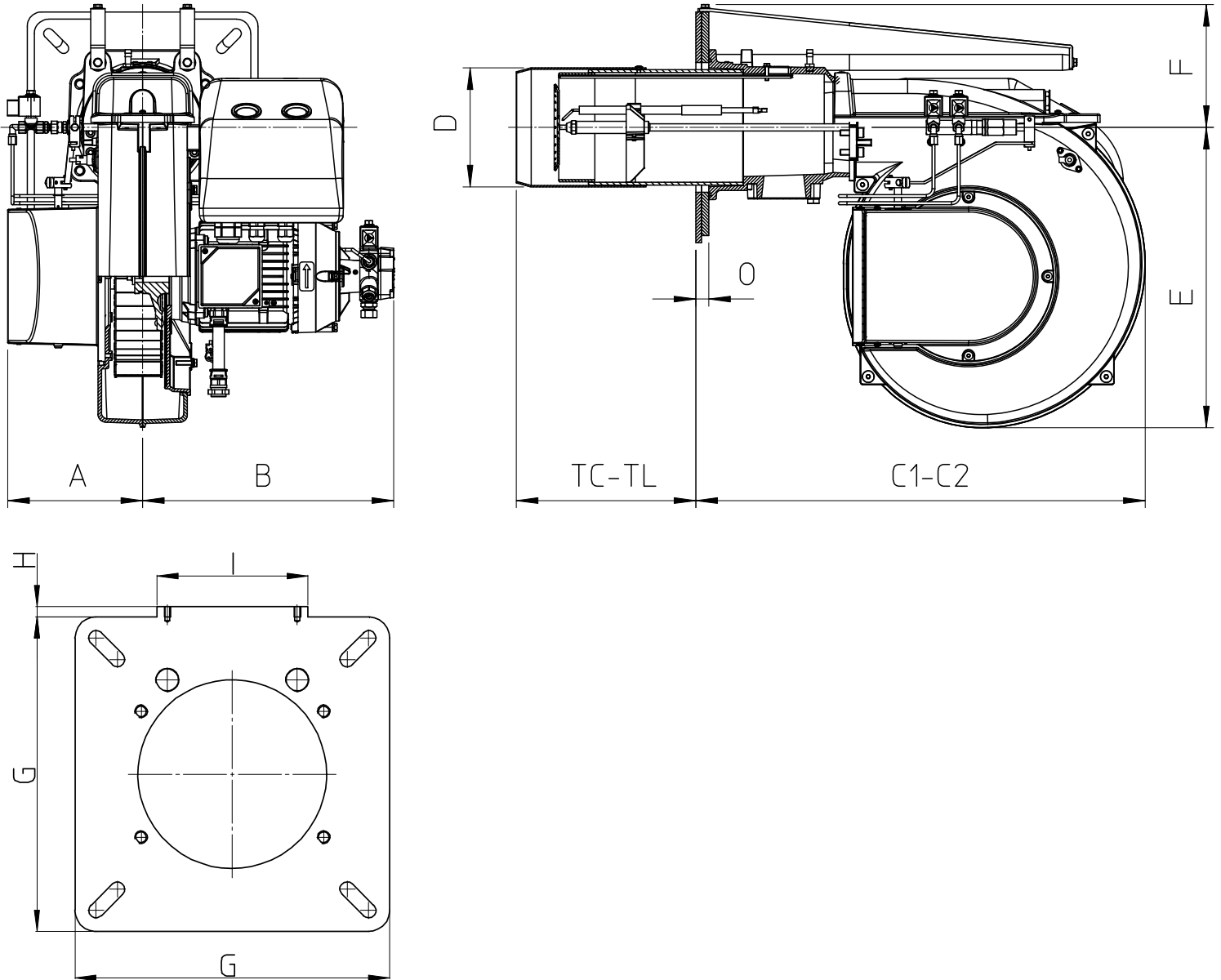
Fig.3 Medidas FGP 75/2
