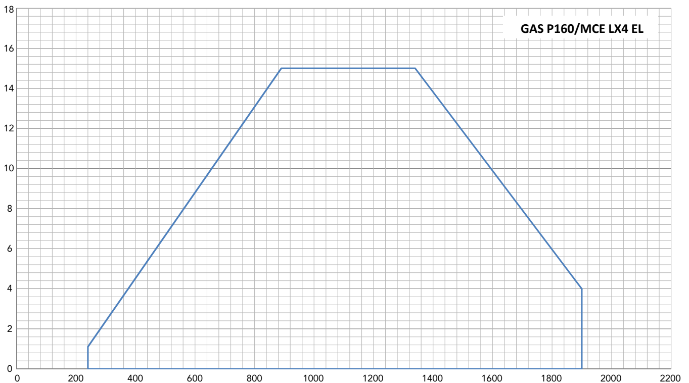
Fig. X = Puissance [kW] Y = Pression en chambre de combustion [mbar]
