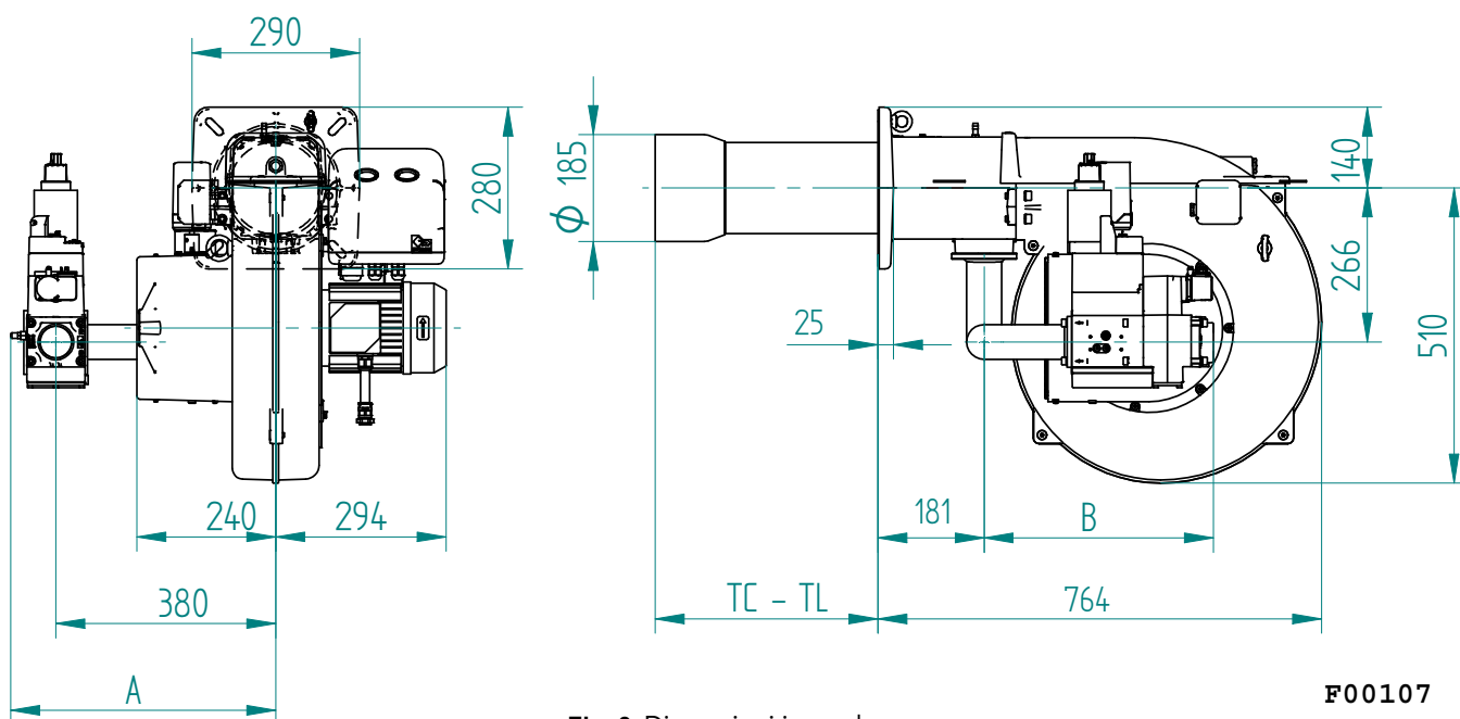
Fig. 3 Dimensioni ingombro
