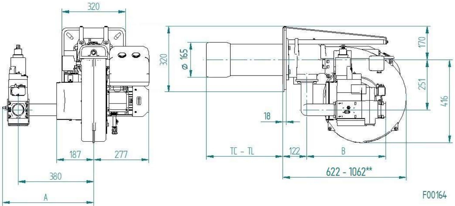
Fig. 3 Dimensioni ingombro
