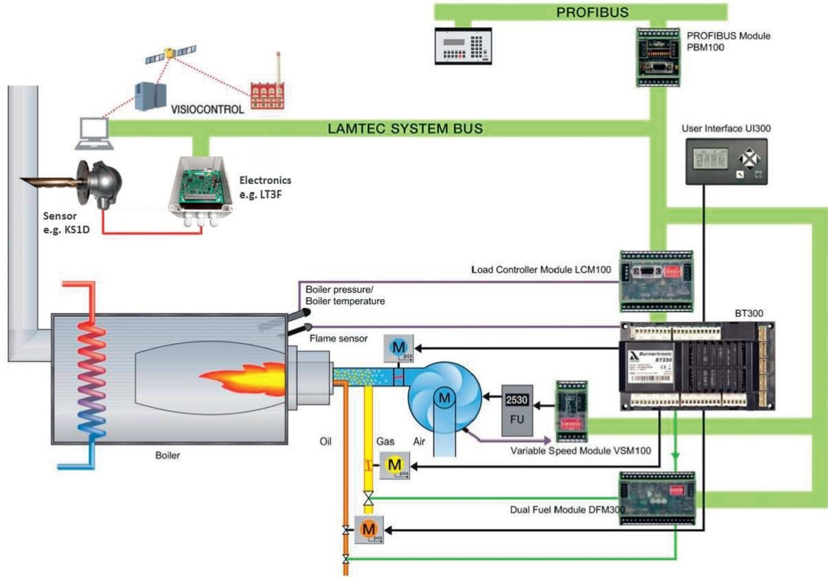
Fig. 2 Cam électronique Lamtec BT3
