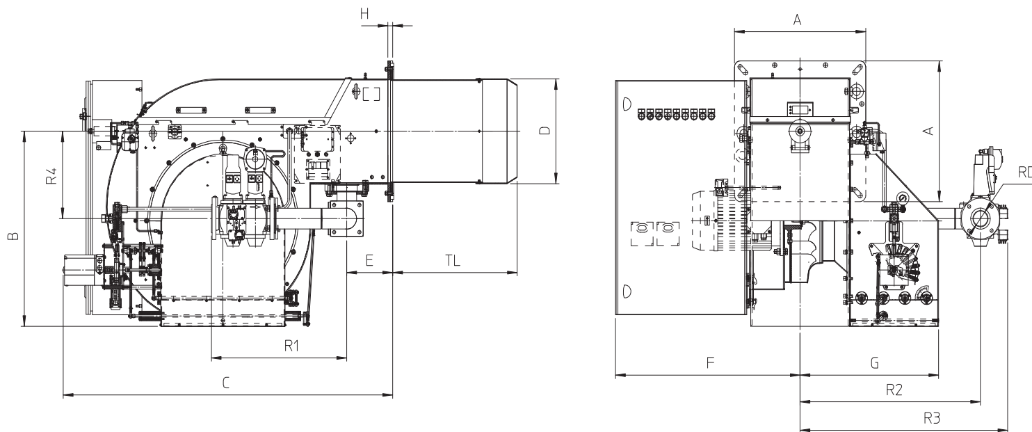
Fig. 5 Dimensions
