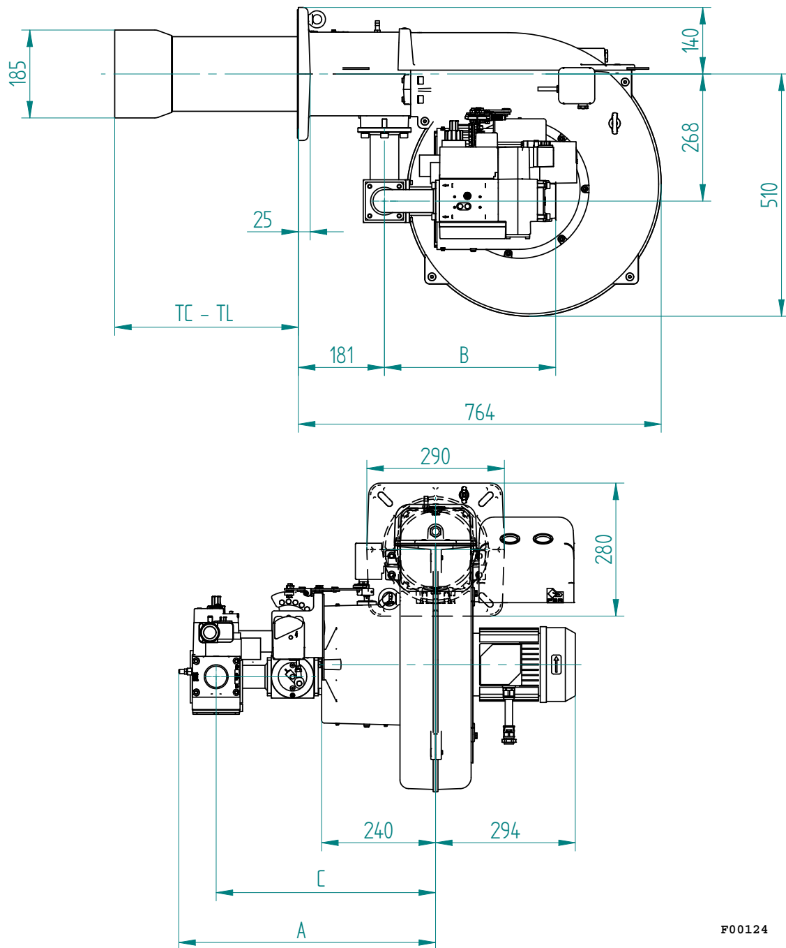
Fig. 3 Dimensioni ingombro
