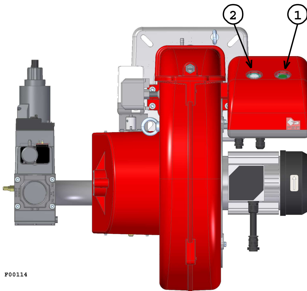
Fig. 4 Segnalazioni bruciatore
