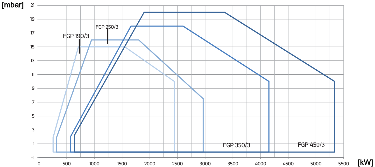
Fig. 2 X = Potencia Y = Presion en camara de combustion
