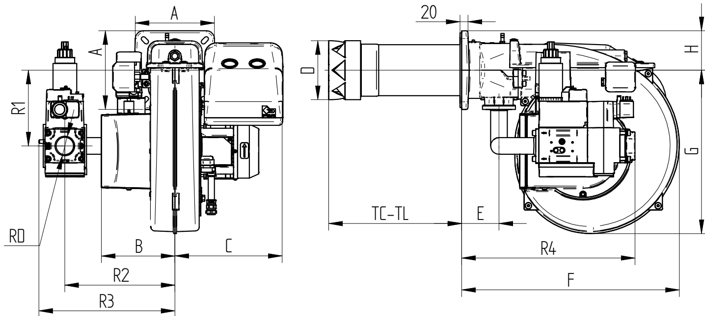
Fig. 2 РАЗМЕРЫ
