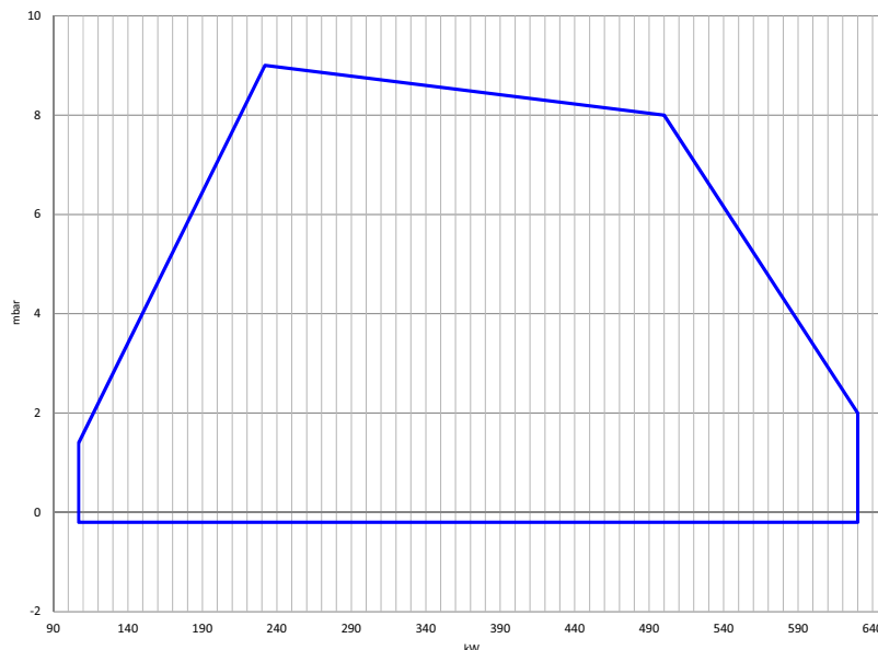
Fig. 2 X = Puissance Y = Pression en chambre de combustion
