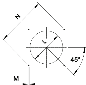
Fig. 3 Pletina de fijación del quemador
