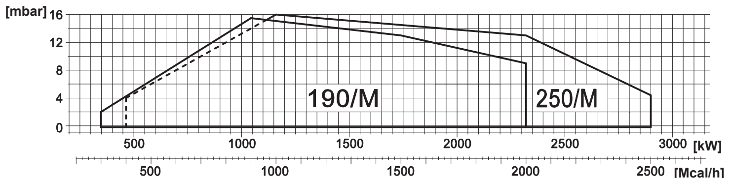
Fig. 2 X = Puissance (kg/h - Mcal/h) Y = Pression en chambre de combustion (mbar)
