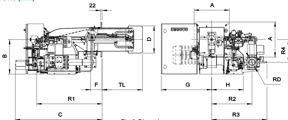
Fig. 3 Dimensions
