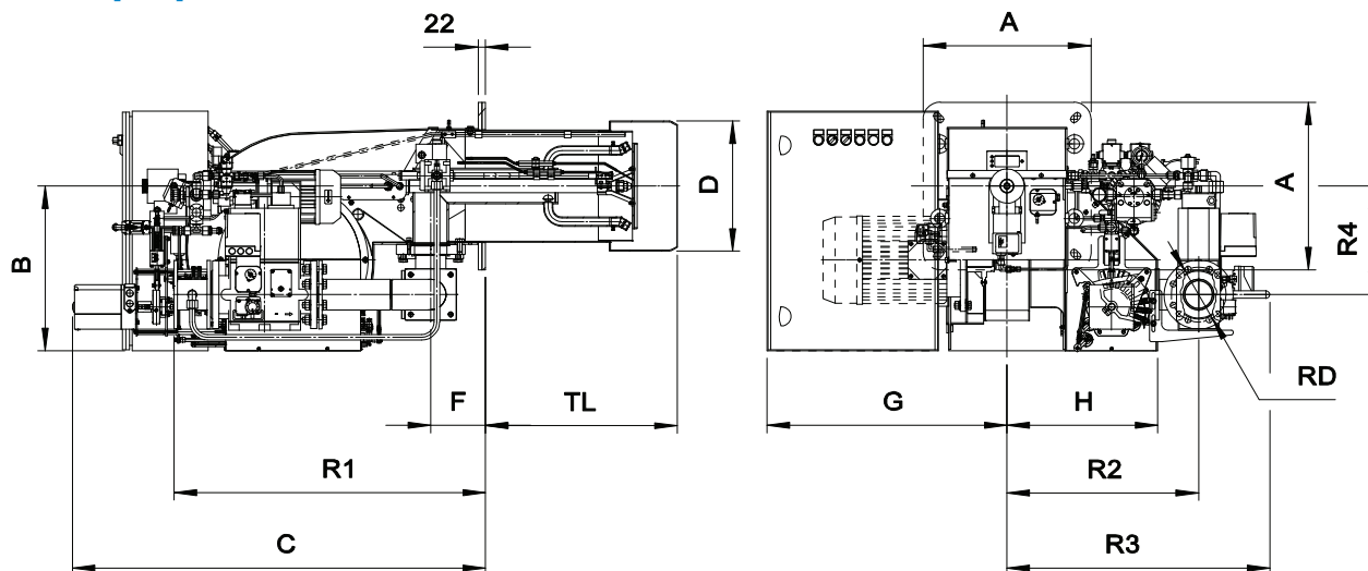
Fig. 3 Dimensioni ingombro
