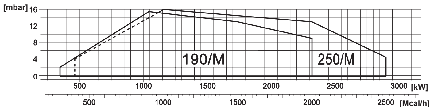
Fig. 2 X = Potenza termica Y = Pressione in camera di combustione
