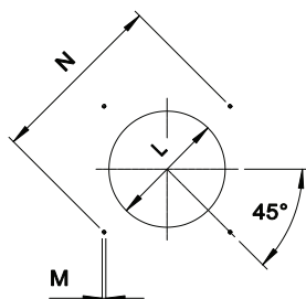
Fig. 4 Flangia fissaggio bruciatore
