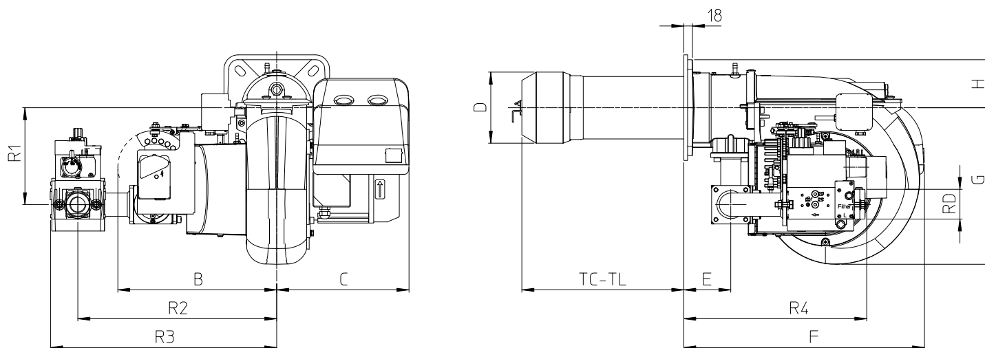
Fig. 3 Dimensions
