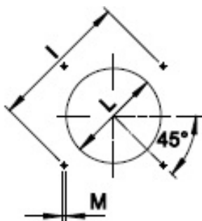
Fig. 4 Plaque porte-brûleur
