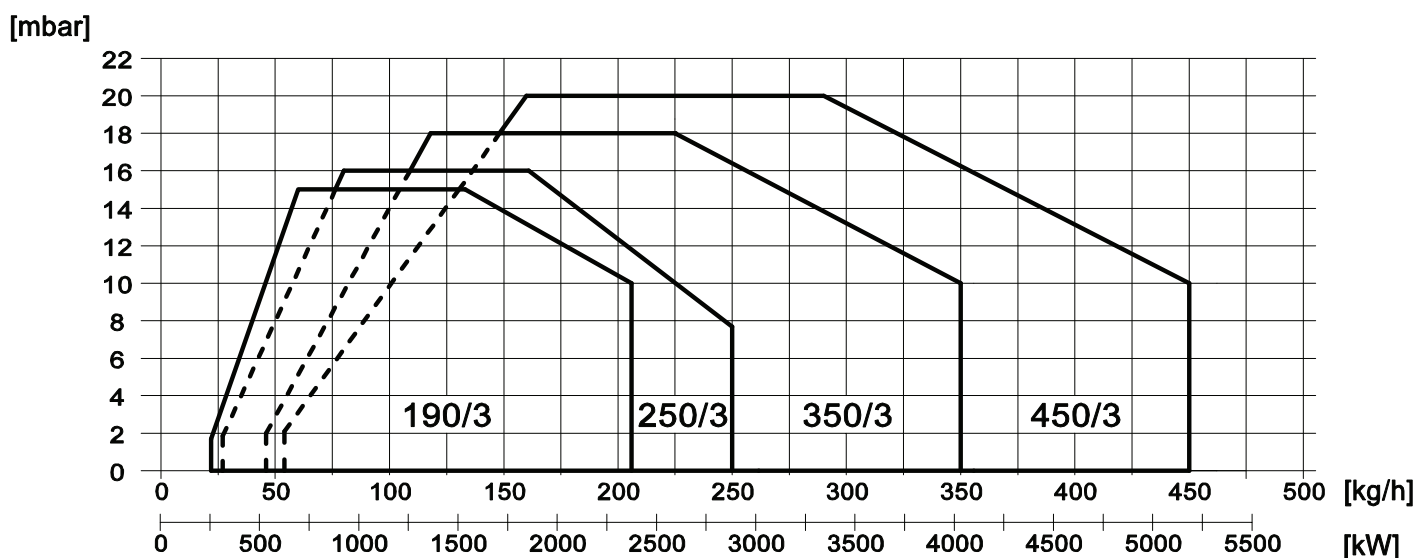
Fig. 2 X = Puissance Y = Pression à la chambre de combustion
