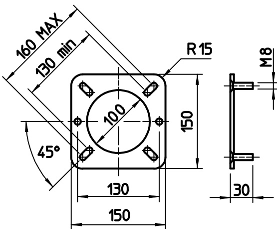
Fig. 4 Pletina de fijación del quemador
