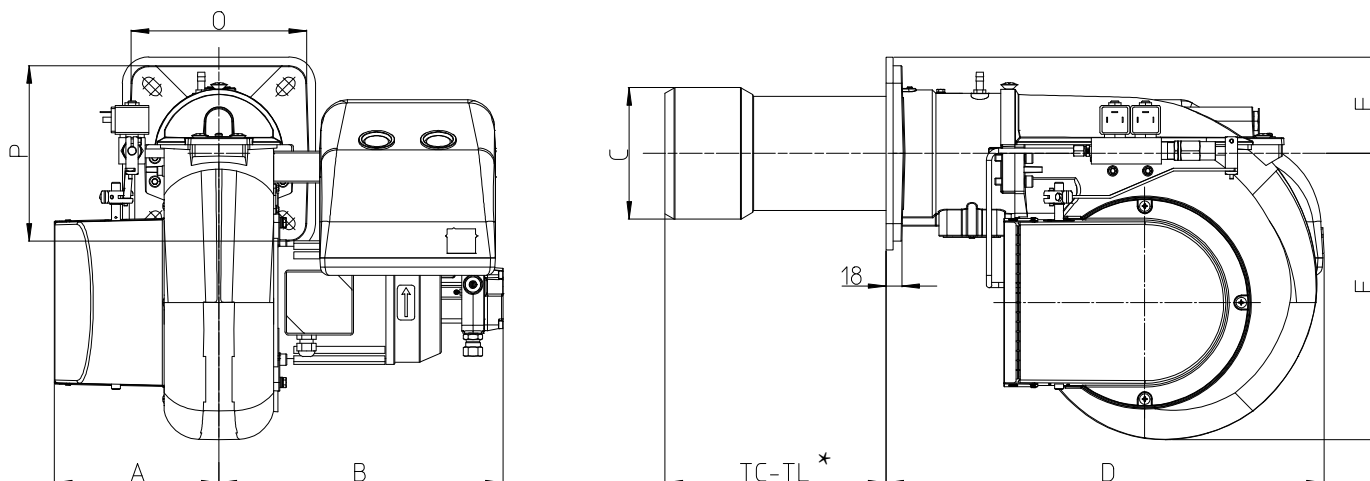
Fig. 5 Medidas FGP 50/2
