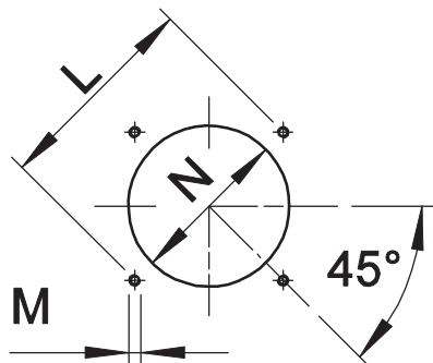
Fig. 5 Plaque porte-brûleur
