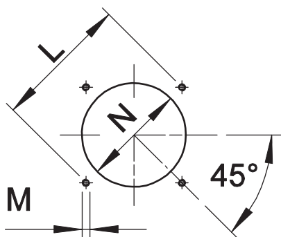
Fig. 5 Pletina de fijación del quemador
