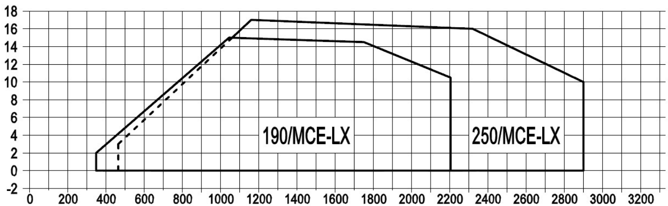
Fig. 1 X = Portata (kW) Y = Pressione in camera di combustione (mbar)
