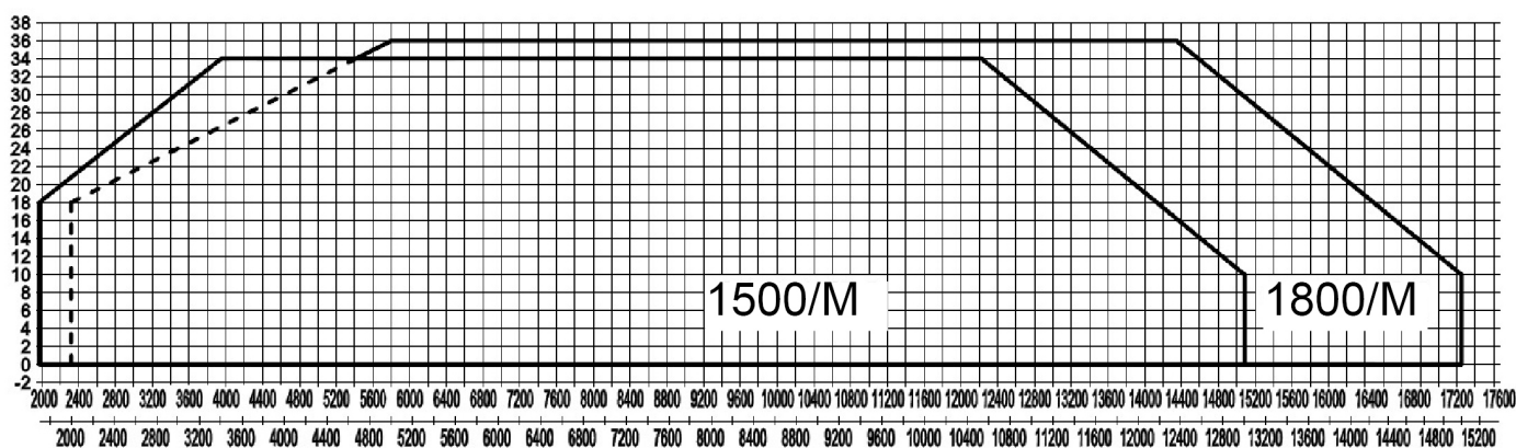
Fig. 2 X = Portata (kg/h - Mcal/h) Y = Pressione in camera di combustione (mbar)
