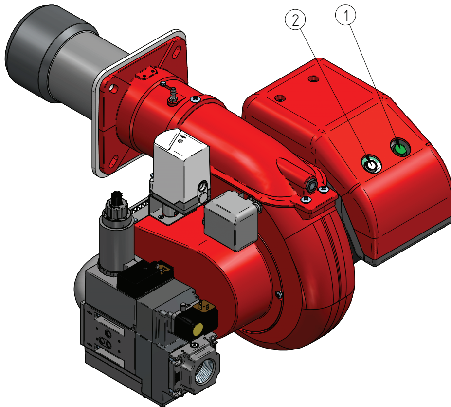
Fig. 5 Segnalazioni bruciatore
