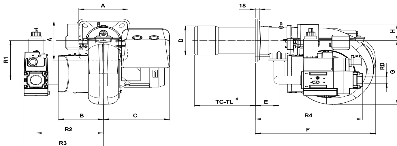
Fig. 3 Dimensioni ingombro GAS XP60/2 CE
